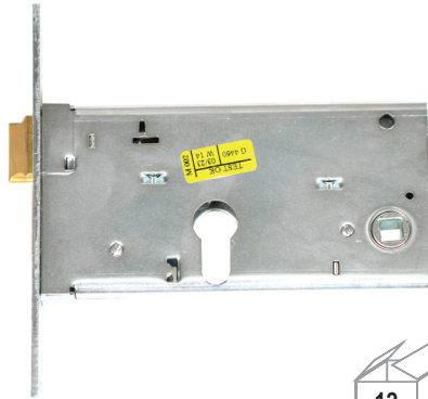
4311 Belgi lock 4300 زر فيل ٤٣٠٠ عرضي
